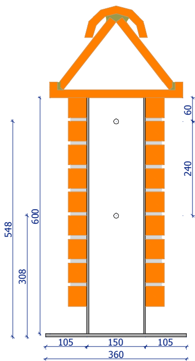
SEZIONE
