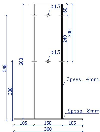
SEZIONE
