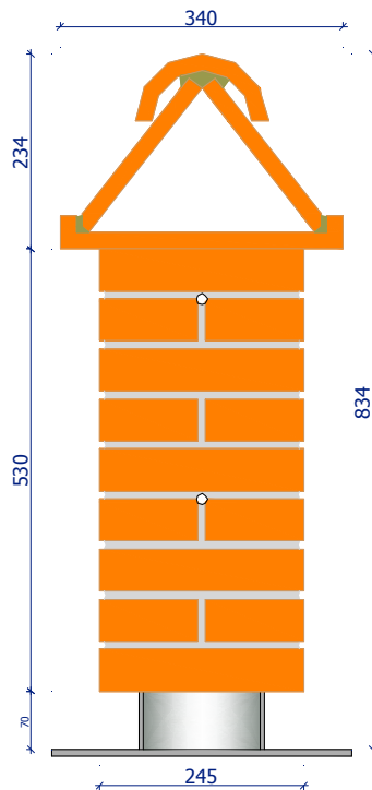
PROSPETTO
